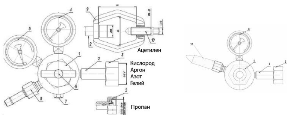
Рис. 1. Редуктор.
