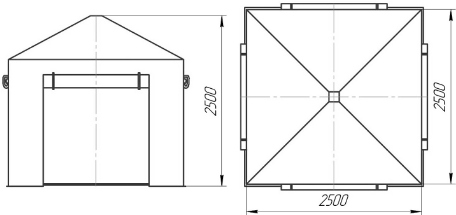
Рис. 1. Общий вид палатки сварщика.
