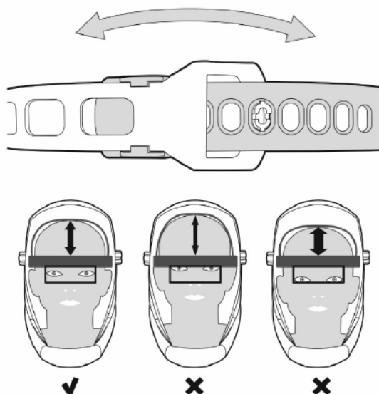
Рис. 8.5. Вертикальная регулировка.
