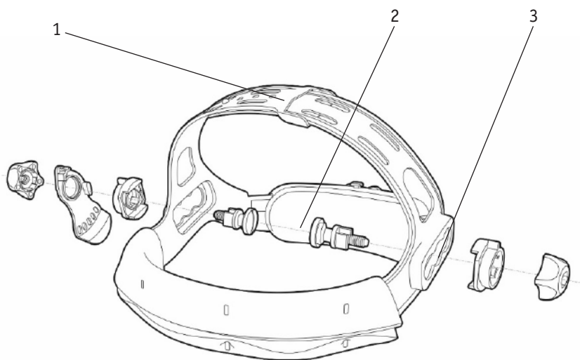
Рис. 8.0.2. Степени свободы наголовника.
