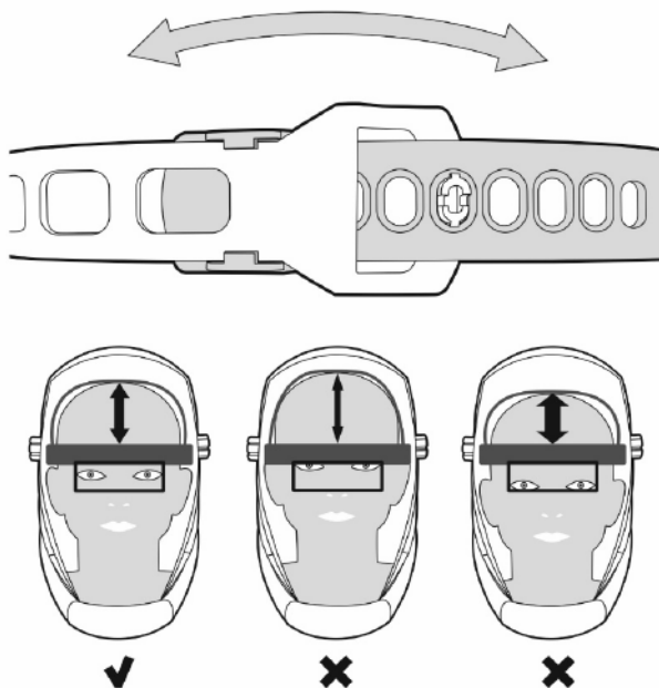
Рис. 8.2.2. Вертикальная регулировка.
