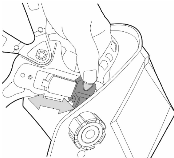
Рис. 8.3.1. Регулировка «ближе/дальше».
