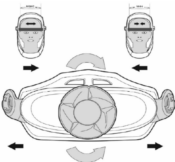
Рис. 8.2.1. Горизонтальная регулировка.
