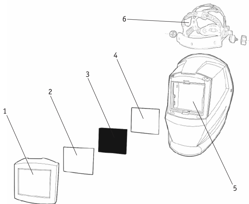
Рис. 7.0.1. Внешний вид.
