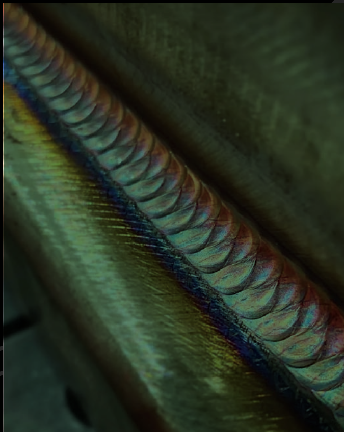
Так видит сварщик через обычный светофильтр-хамелеон
