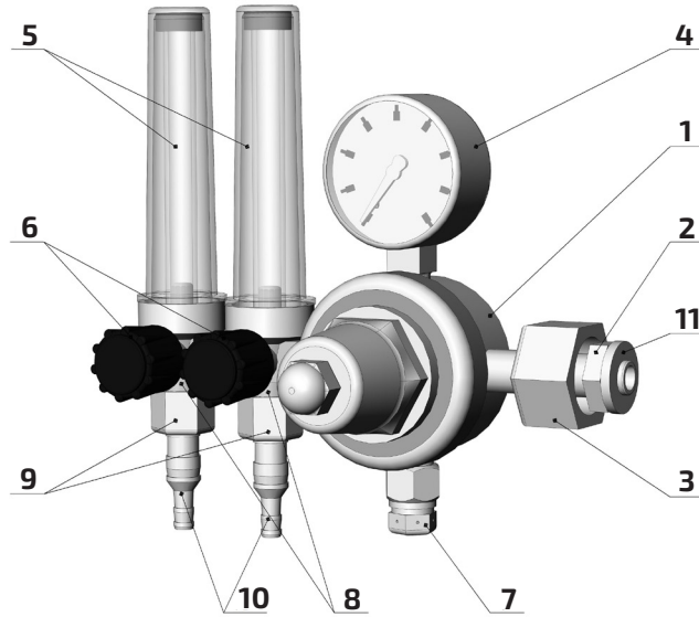
Рис. 1. Регуляторы расхода газа.
